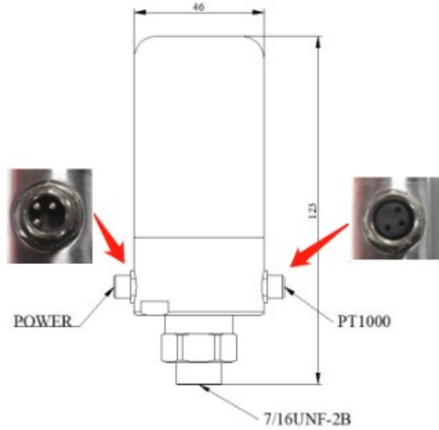
图 1 外形图
