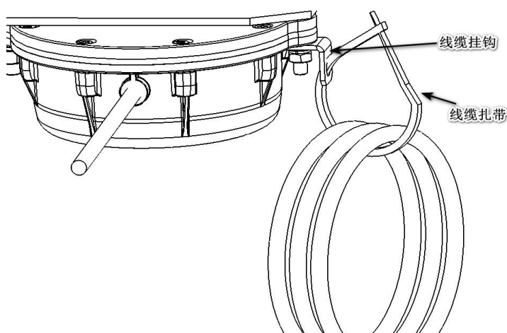
图4 线缆绑扎示意图 (安装附件 CS-iTWM-05D-A02)
