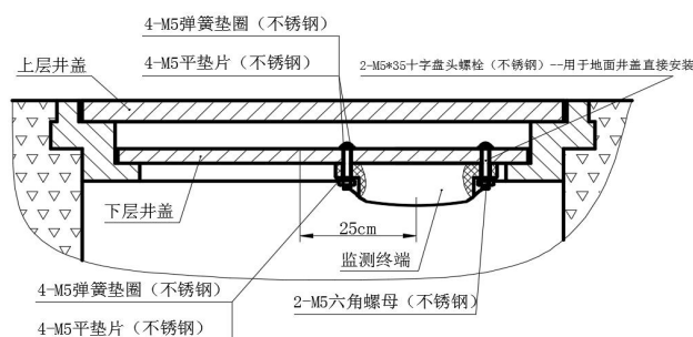
图3 打孔安装示意图 (安装附件 CS-iTWM-05D-A02)
